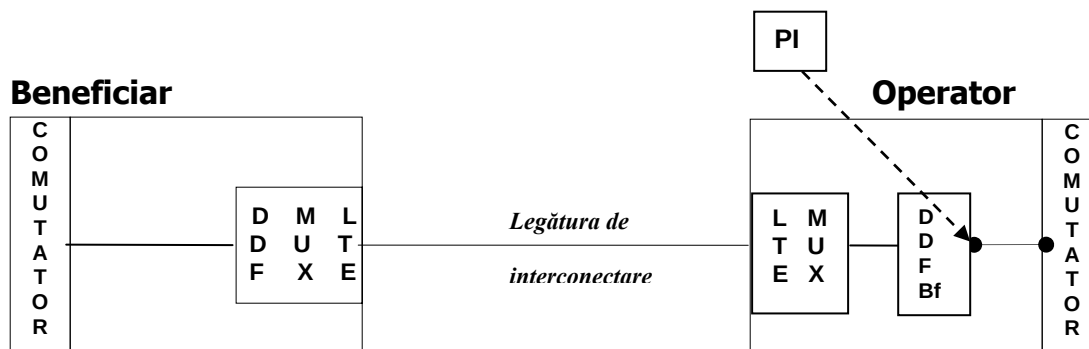
Figura 3 – Interconectare directă în spațiul Operatorului (exemplu)
