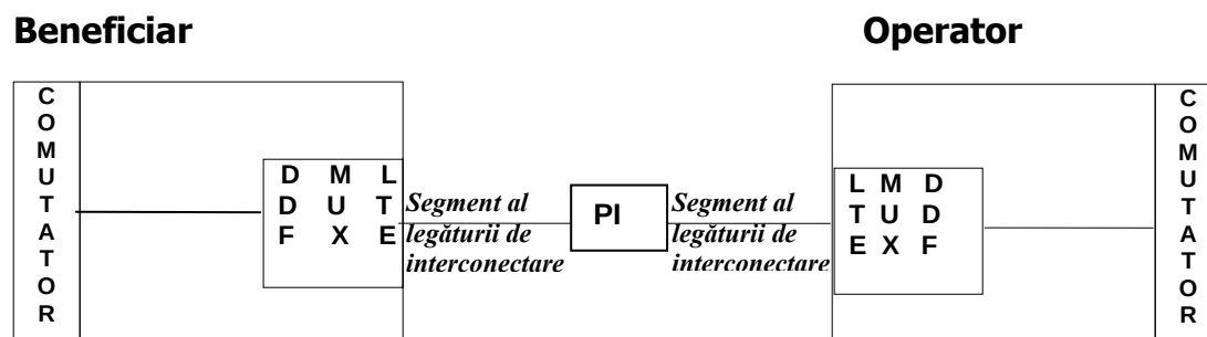
Figura 2 – Interconectare directă la un punct intermediar (exemplu)
